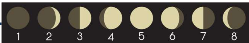
Schéma des phases de la Lune
